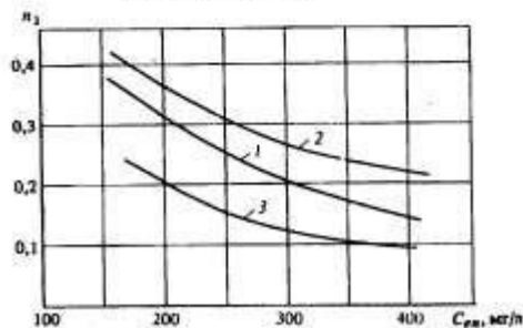
Черт. 2. Зависимость показателя степени n_2 от исходной концентрации взвешенных веществ в городских сточных водах при эффекте отстаивания 1 – \Delta = 50\% ; 2 – \Delta = 60\% ; 3 – \Delta = 70\%
